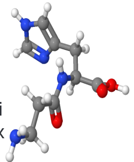
Structure 3D de la Carnosine
