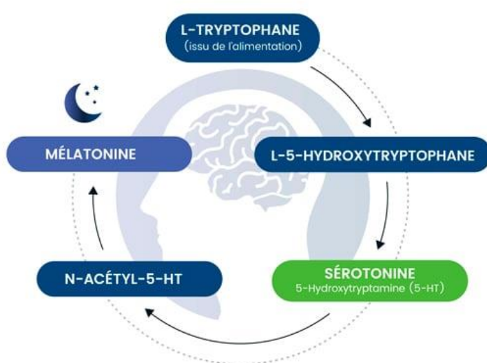
Biosynthèse de la sérotonine et de la mélatonine
